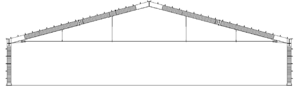
Uddevalla 2 (single tension bar)
