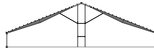
RAMTYP: GDANSK FÖR STÖRRE BYGGNATIONER MED MITTGÅNG
